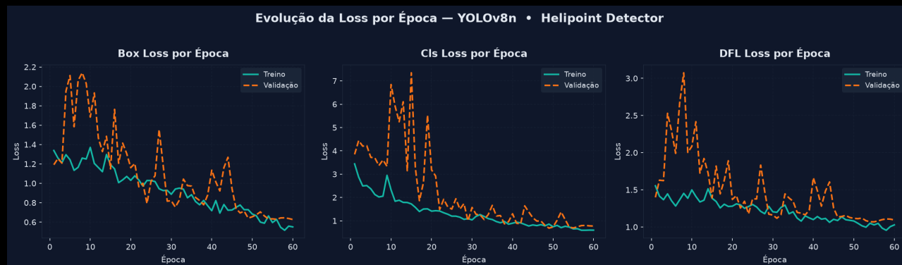
Figura 1 — Evolução das Losses por Época
