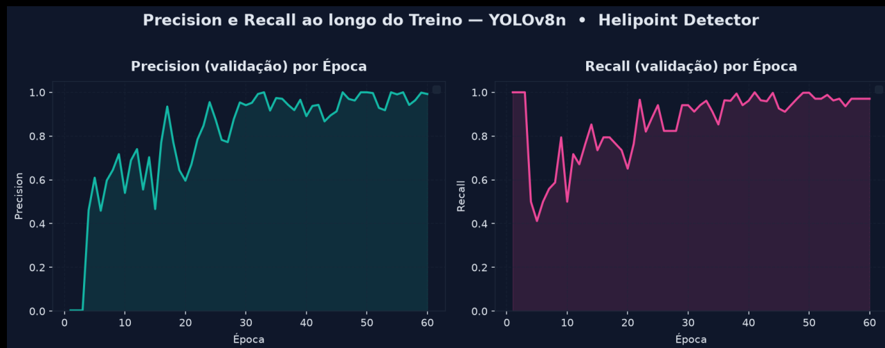
Figura 2 — Precision e Recall ao Longo do Treino
